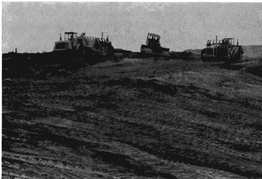
To meget store grave- og transportmaskiner suppleret af en bulldozer (i midten) arbejder med fjernelse af overjord i brunkulsleje i Søby. Hver af maskinerne tager 10 tons ad gangen. Der skal flyttes 600.000 m 3 overjord, inden det nye leje kan tages i brug, fot. maj 1963.
